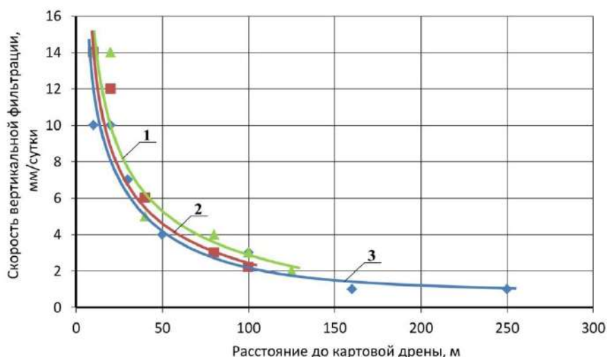
Рис.1. Скорость вертикальной фильтрации на картах-чеках в зависимости от расстояния между дренажными каналами: 1 – В = 200 м; 2 – В = 250 м; 3 – В = 500 м
